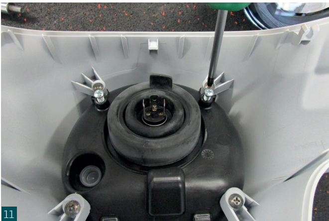
11 Scheinwerfer montieren. Zur Erstmontage die Schrauben mit einem Schmierstoff versehen. Mount headlight. For initial assembly, apply lubricant to the screws.
